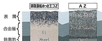
図 1 皮膜構造図
